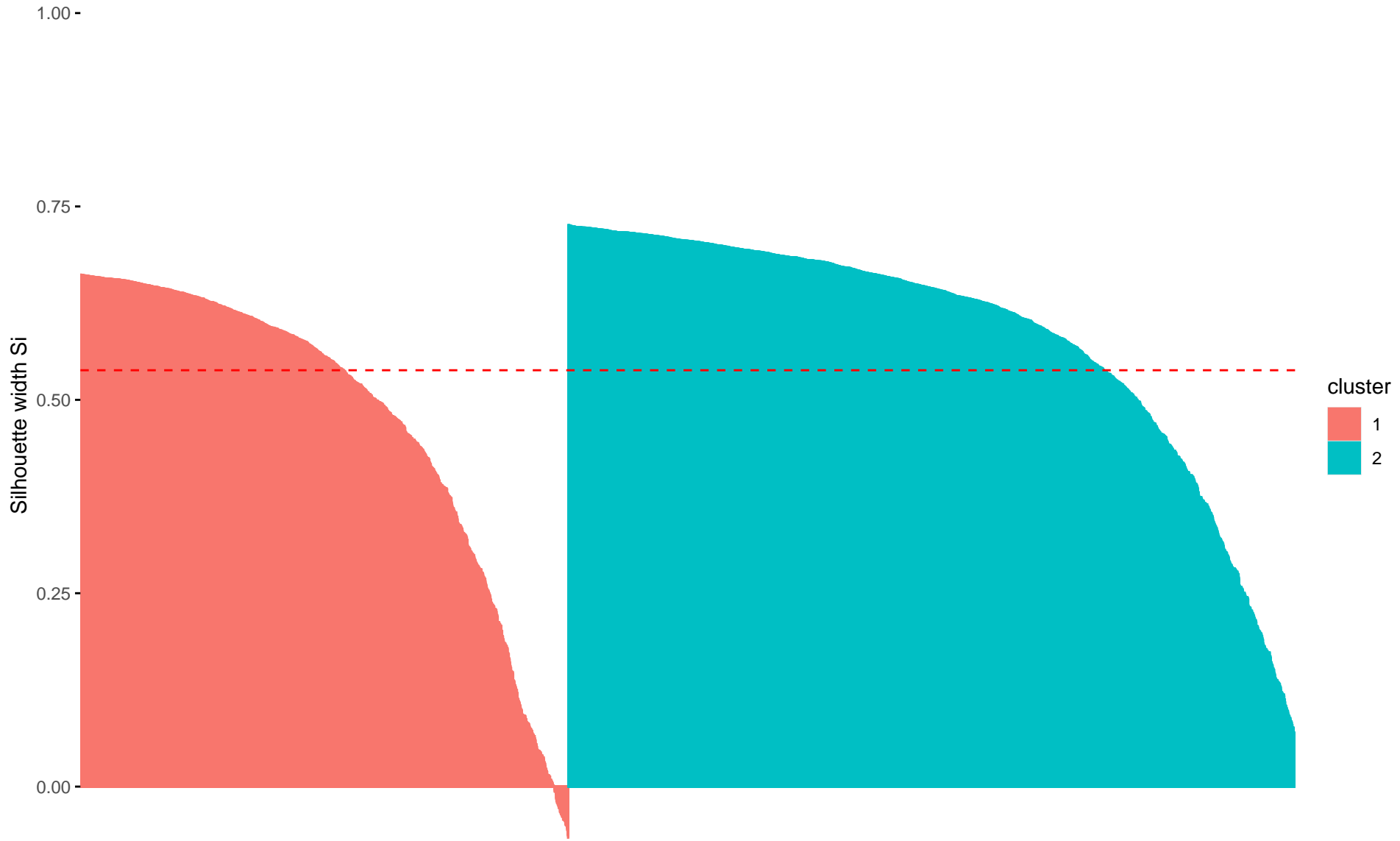
pam silhouette (k=2)
